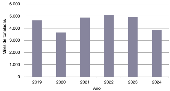
Producción de acero crudo
