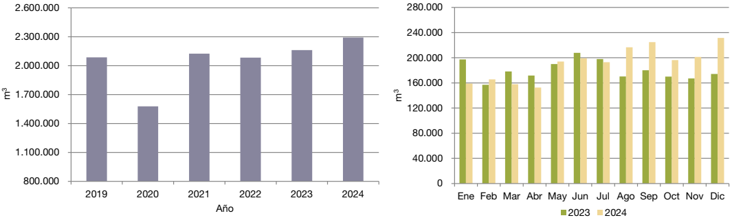
Producción de nafta especial premium > 97 RON
